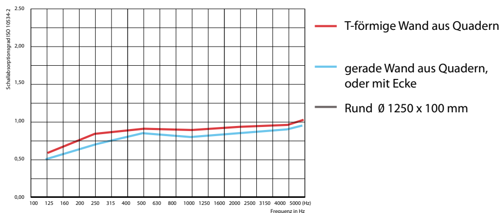
Schallabsorptionsgrad der Elemente (nach Herstellerangaben)
